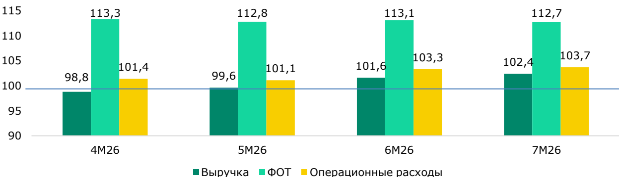
Рис. 2. Структура HBI
