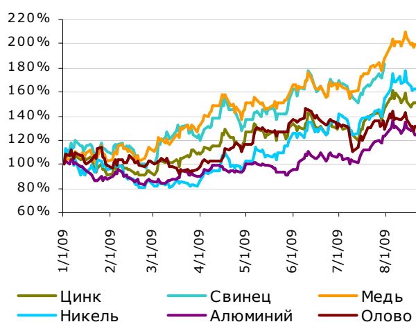
Рисунок 1. Резкая коррекция после пика 2009 года, ЛБМ (цены индексированы на 1 января 2009г.)
