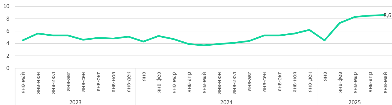
Рис.1. Динамика КЭИ, %
